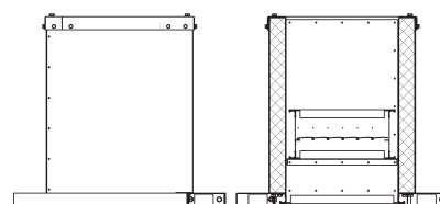
СМ.1 Стакан с утеплением и АВК
