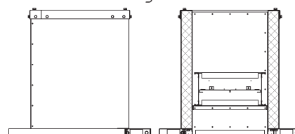
СМ.1 Стакан с утеплением и ПК
