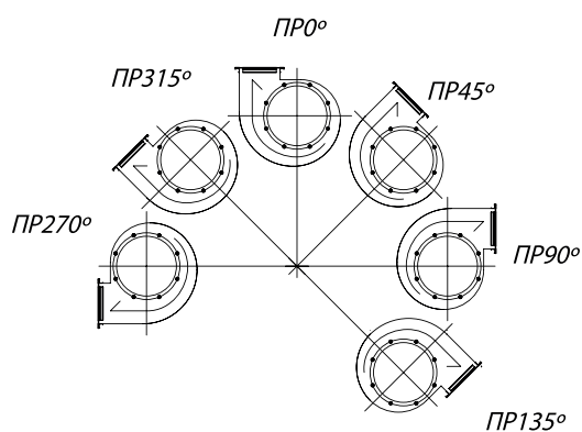
Положение корпуса вентилятора радиального ВР.280-46 (Вид со стороны всасывающего патрубка)
