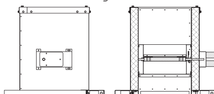
СМ.1 Стакан с утеплением и ППШ
