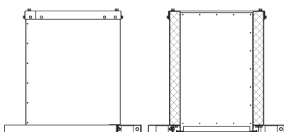
СМ.1 Стакан с утеплением
